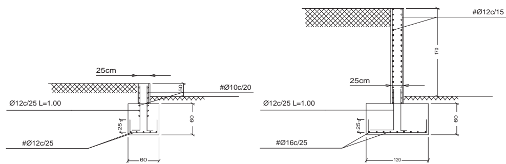
MURO HORMIGÓN. TRAMO 1- DESDE 0,50 m HASTA 1,20 m.
