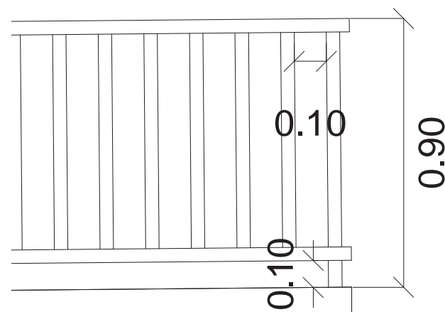
BARANDILLA esc 1/20
